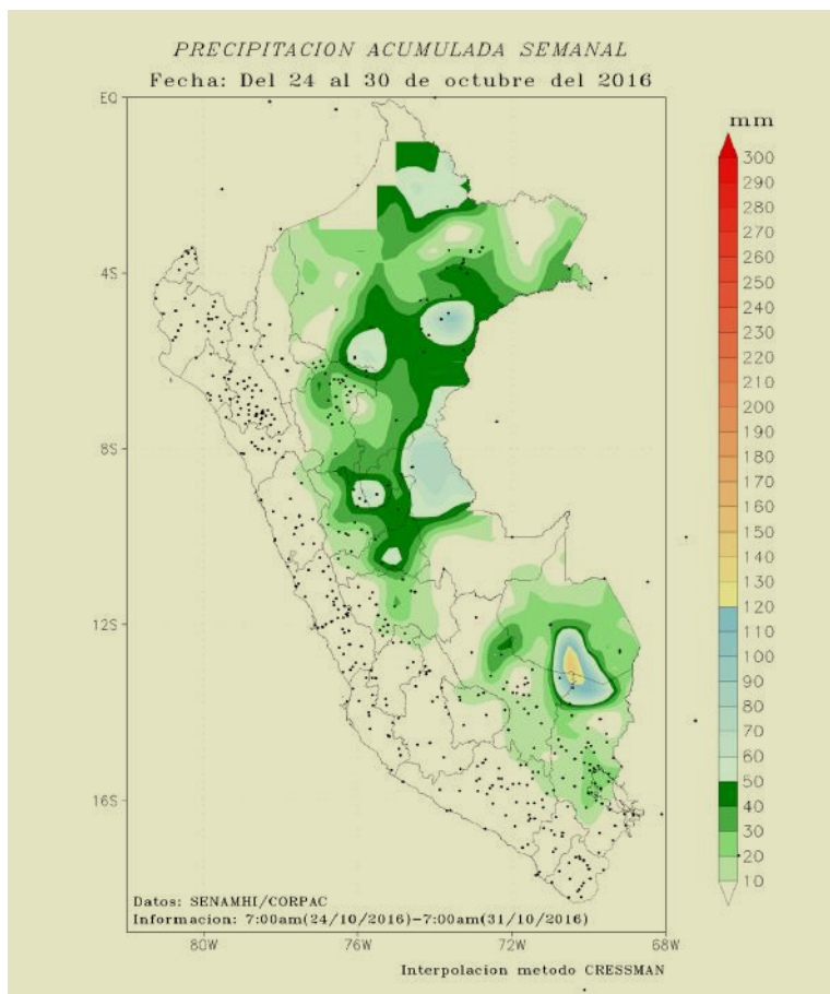
Mapa N° 3 Promedio semanal de precipitación acumulada del 24 al 30 de Octubre del 2016
