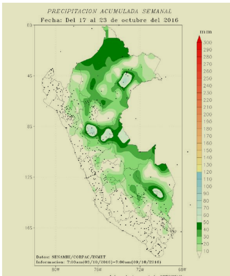
Mapa N° 2 Promedio semanal de precipitación acumulada del 17 al 23 de octubre de 2016
